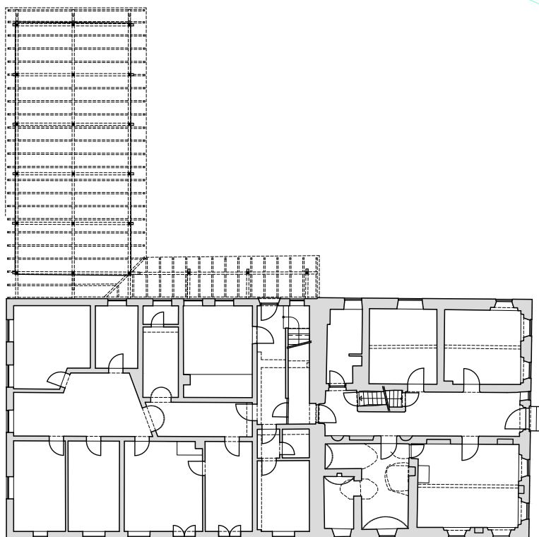
GRUNDRISS EG UND ANSICHT OST KAUMHOF • BERGEN AUSWERTEMAßSTAB M=1:50 (Aufmaß durch Laserscanning)
